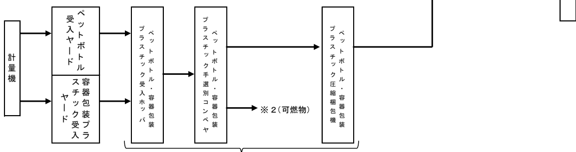
図 5-1 ごみ種類別処理フロー (1/2)
