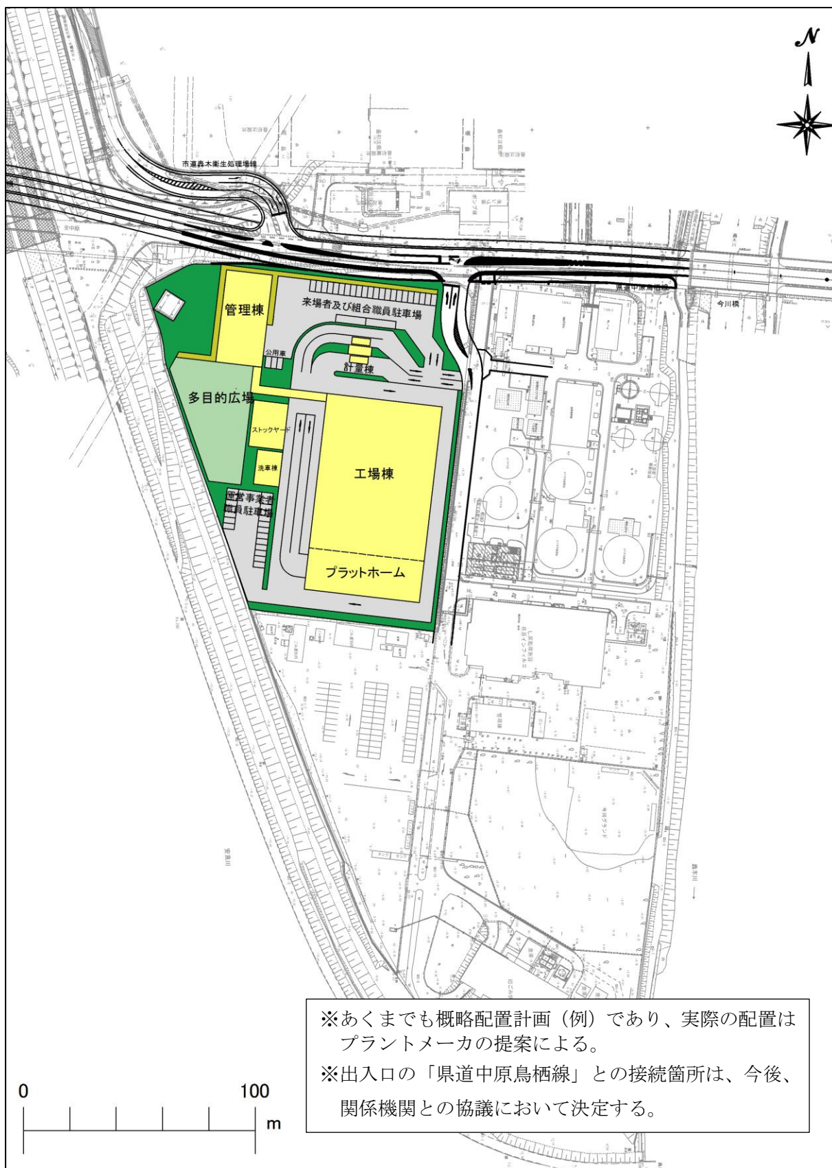
図6 概略配置計画（例）
