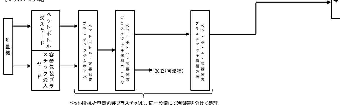
図 3 ごみ種別処理フロー (1/2)
