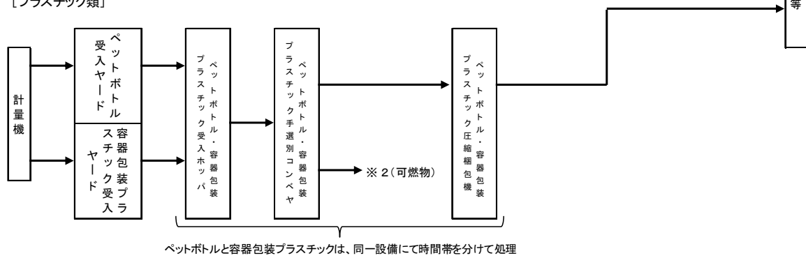
図 5-1 ごみ種類別処理フロー (1/2)
